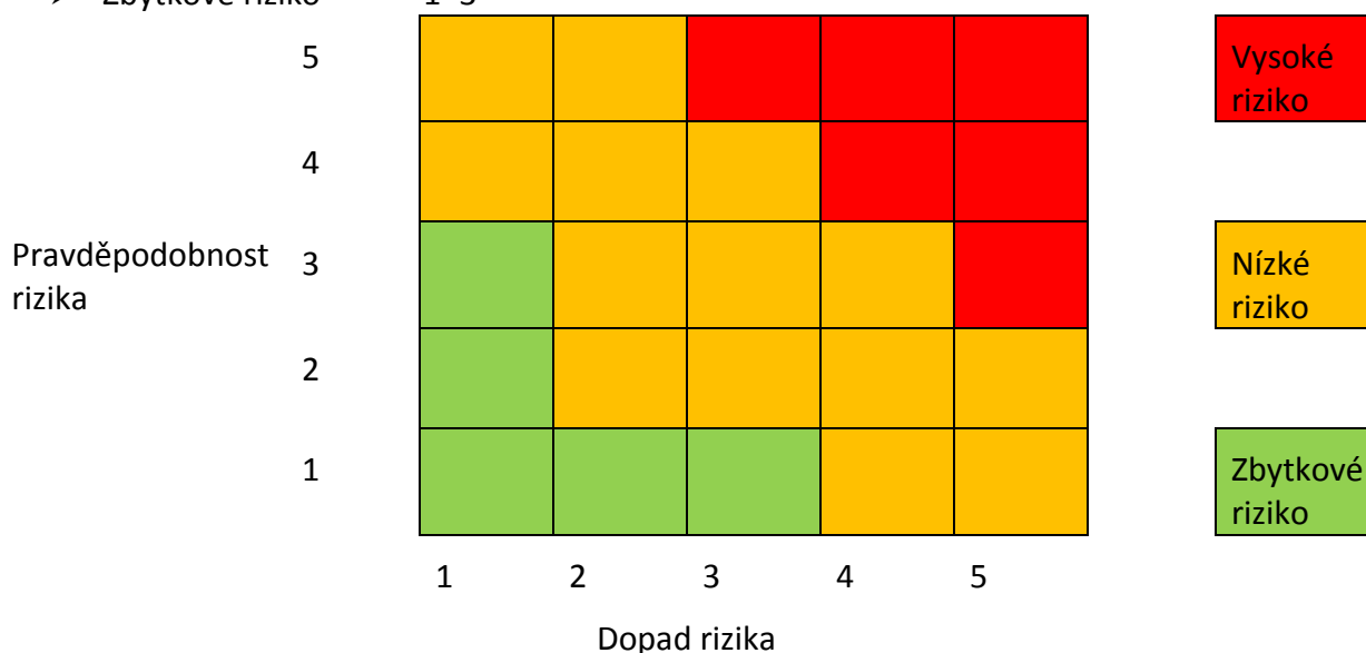
Obrázek 1: Klasifikace rizik
